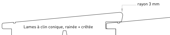
OLWO Profil N° 81
