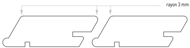
OLWO Profil N° 77
