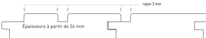
OLWO Profil N° 11+12
