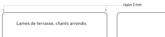
OLWO Profil N° 22
